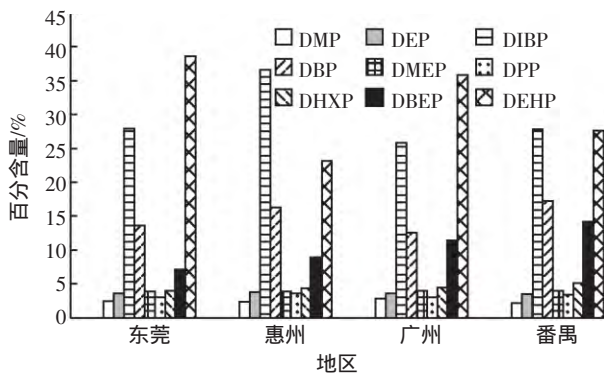
图 1 珠三角地区水稻土壤中单个 PAEs 化合物占 \Sigma PAEs 的百分含量
